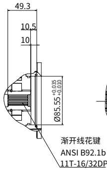
“A2” 型通轴驱动
