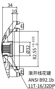
“A2” 型通轴驱动
