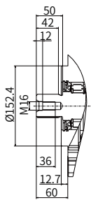
“CE” 型花键轴 DIN 5480 W45×2×21×9 g
