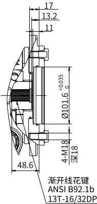
“B1”型通轴驱动
