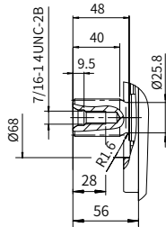
“B4” 型花键轴 ANSI B92.1b 1 1/4 in 14T 12/24DP
