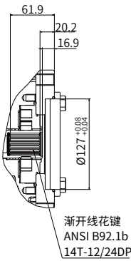
“CC” 型通轴驱动
