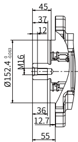
“D4” 型花键轴 DIN 5480 W40×2×18×9g
