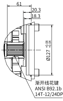
“C2”型通轴驱动
