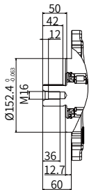
“D5” 型花键轴 DIN 5480 W45×2×21×9g
