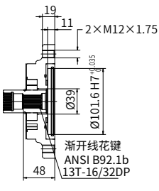
“B1”型通轴驱动
