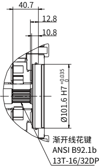
“B1” 型通轴驱动
